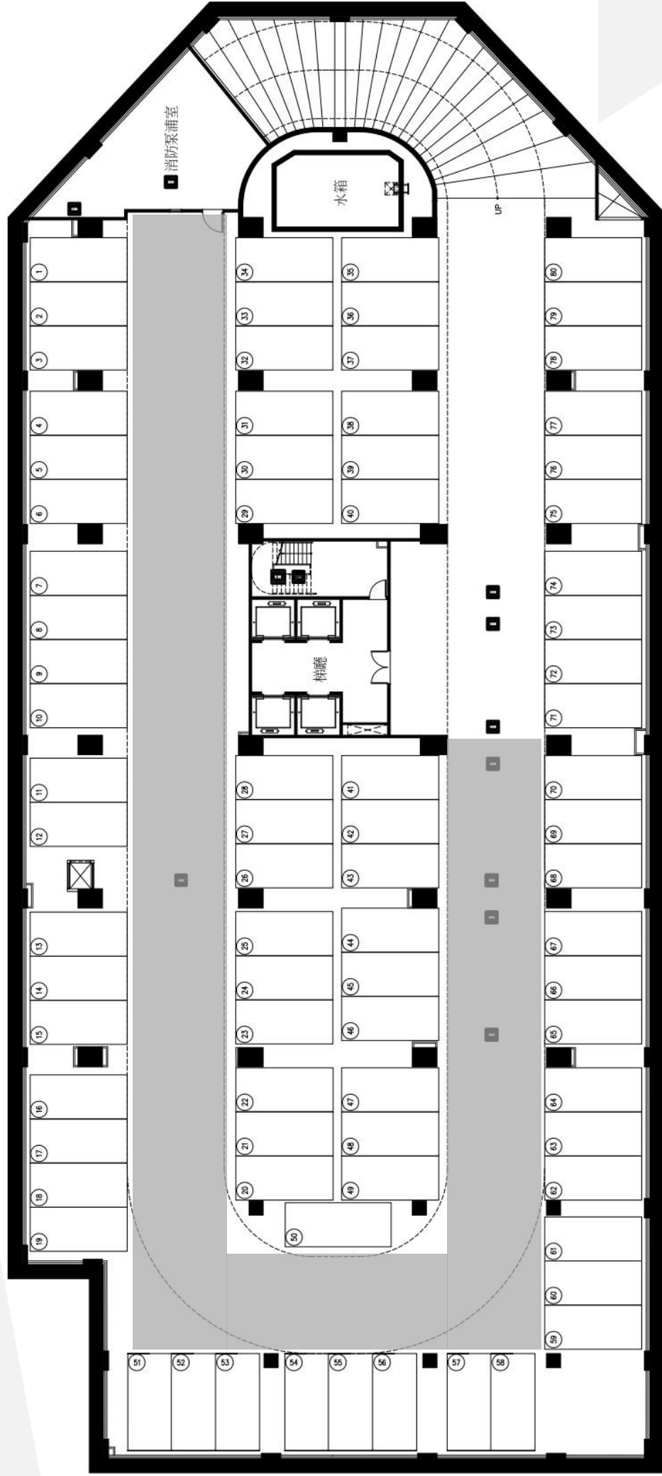
B4 平面配置圖
